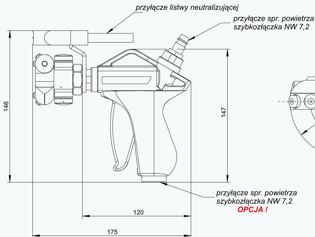
dysza obrotowa model : CRN54-35
